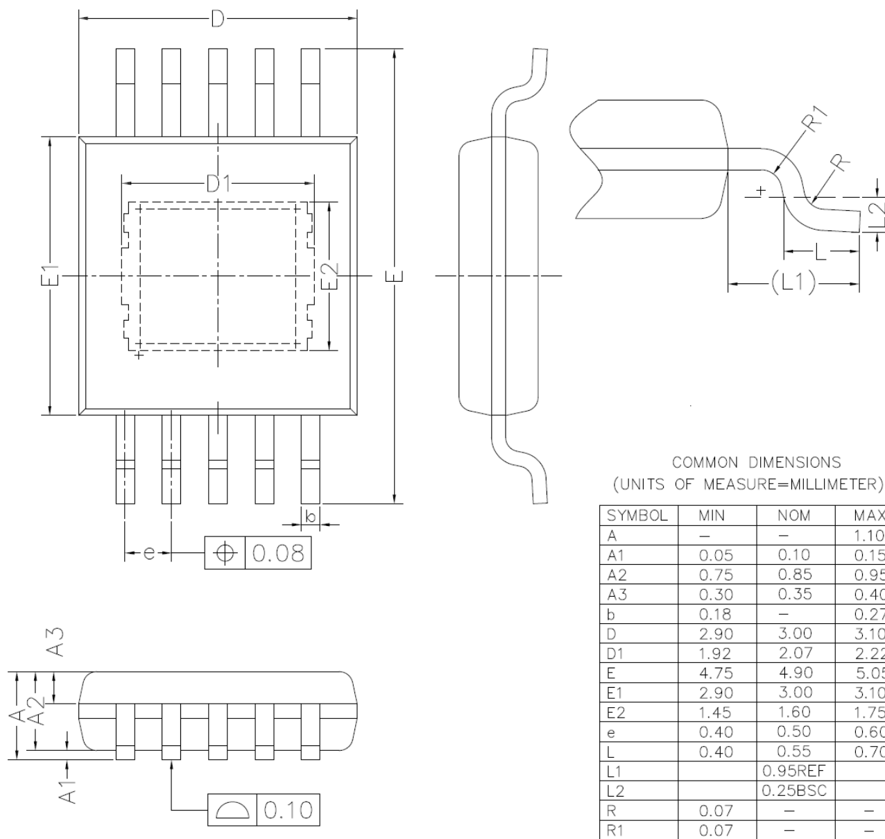
图 24 MSOP 封装
