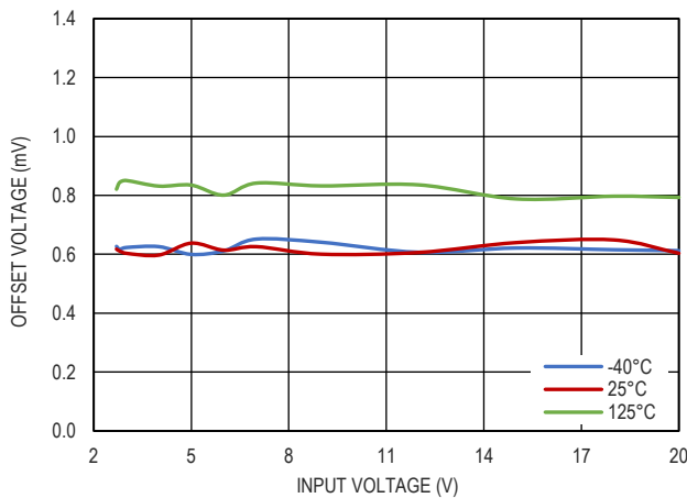
图 7. |V_{OUT} - V_{SET}| 和输入电压的关系, V_{OUT} = 1.8V
