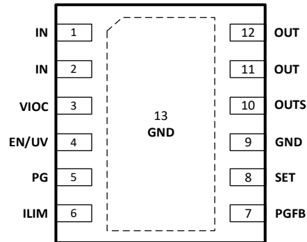
图 3. DFN12 (3mmx3mm GM1205ACPZ-2) 和 PMSOP12 (4mmx4.9mm, GM1205ACPZ-, 兼容 MSOP-12) 引脚配置(顶视图)
