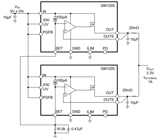
图 24. 并联设备
