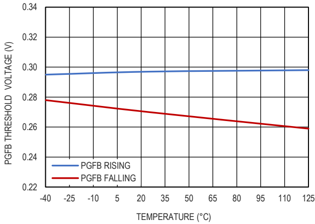
图 17. PGFB pin 阈值
