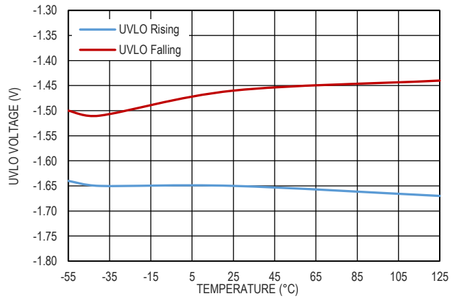
图 12. UVLO 阈值
