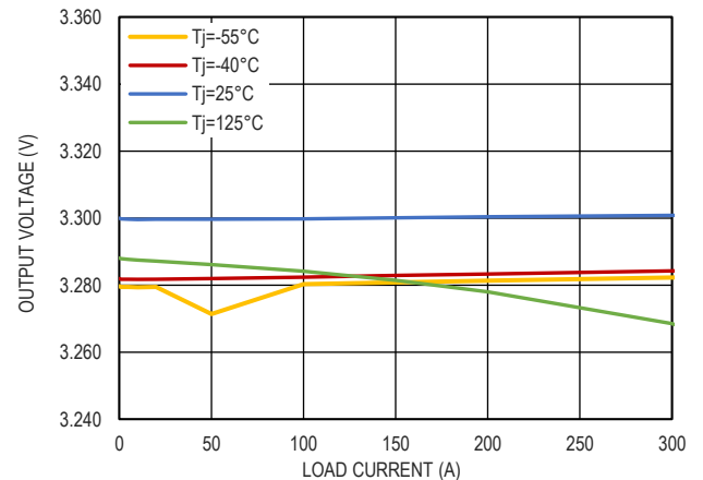
图 12. 3.3V 输出电压和负载电流的关系
