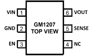
图 5.6 引脚 SOT-23 引脚配置
