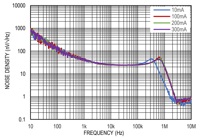
图 18. 输出噪声谱密度, V_{IN}=5V , V_{OUT}=3.3V
