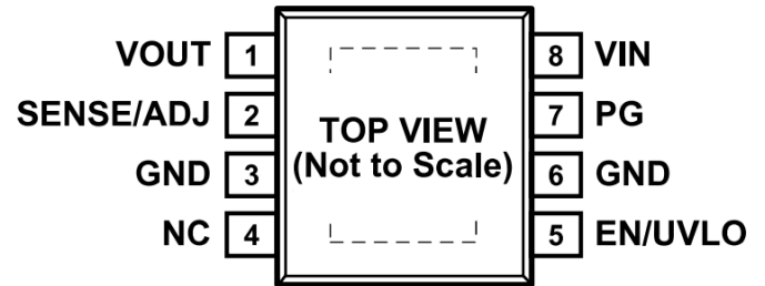
图 6.8 引脚 SOP-8 的引脚配置
