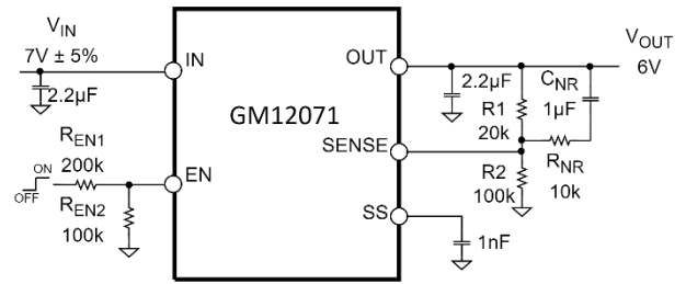
图 30. 噪声优化
