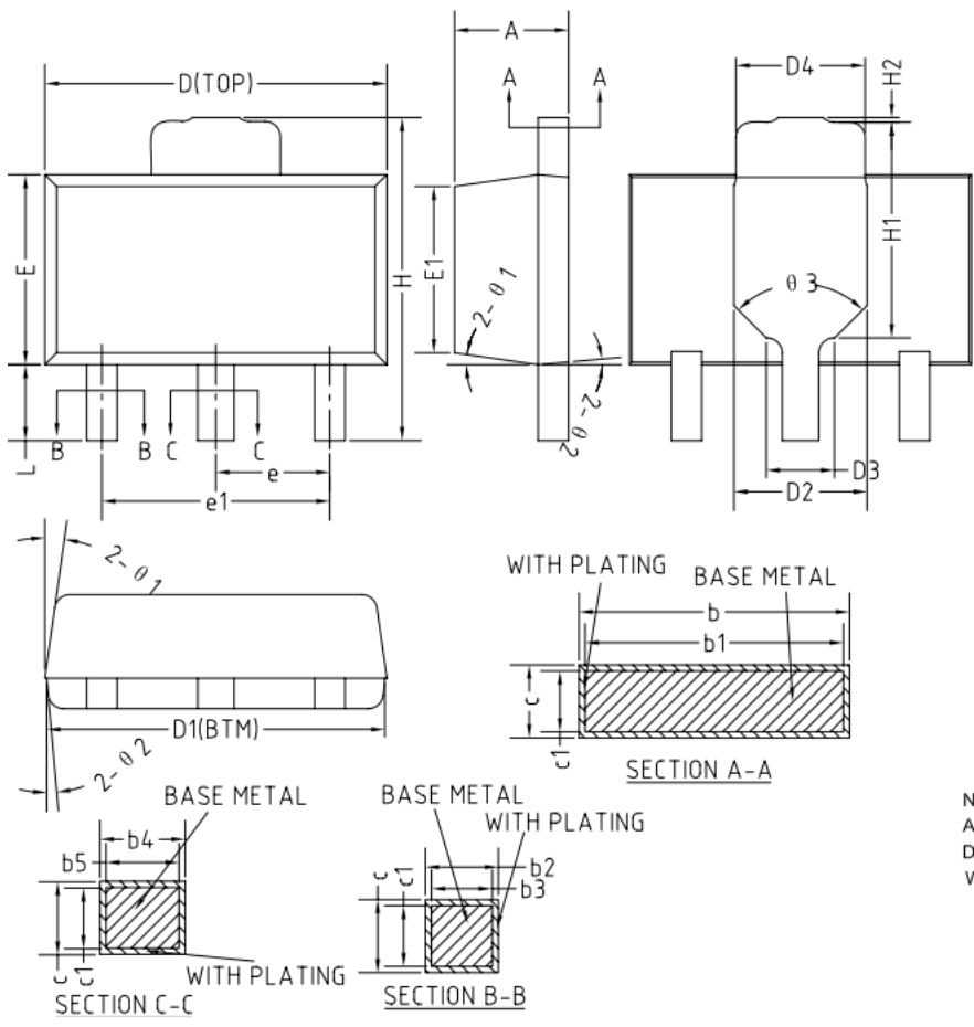
图 37.3 引脚 SOT-89
