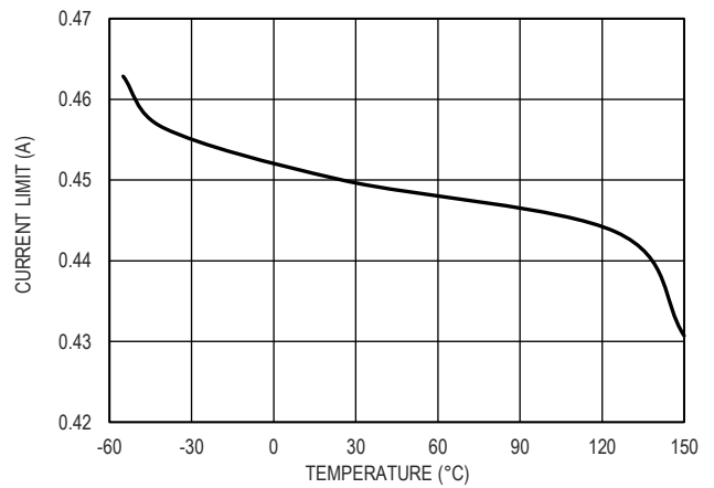
图 17. 输出限流值和温度的关系
