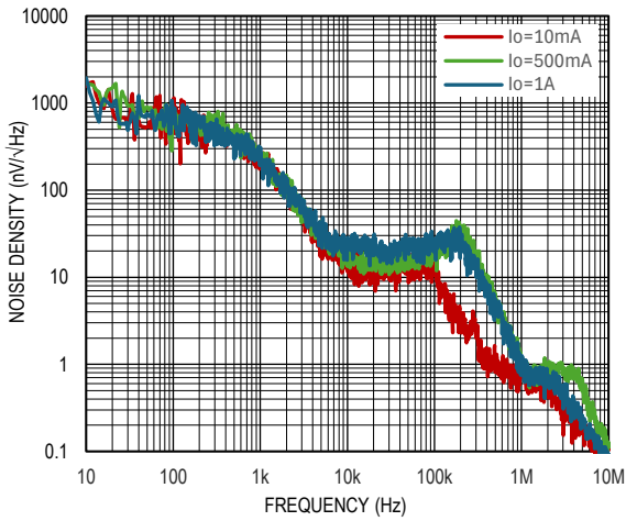
图 9. 噪声谱密度
