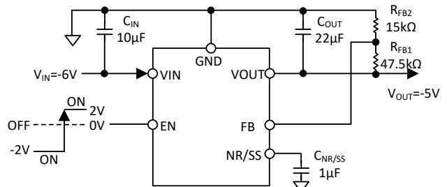
图 17. 设置可调输出电压
