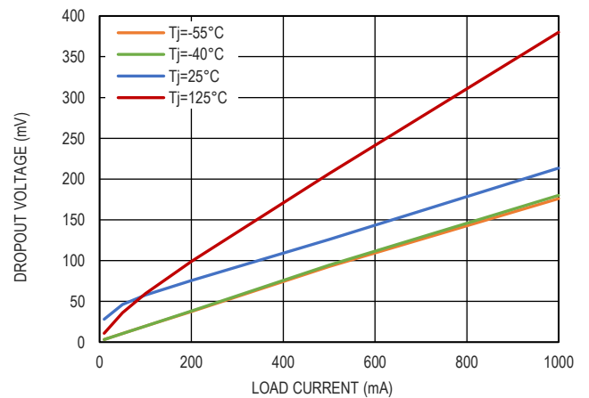
图 8. 压差电压和负载电流的关系
