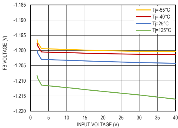
图 5. FB 引脚电压与输入电压的关系
