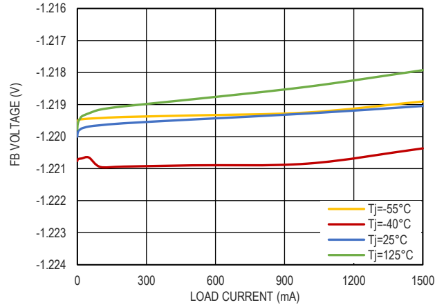
图 5. FB 引脚电压与负载电流的关系
