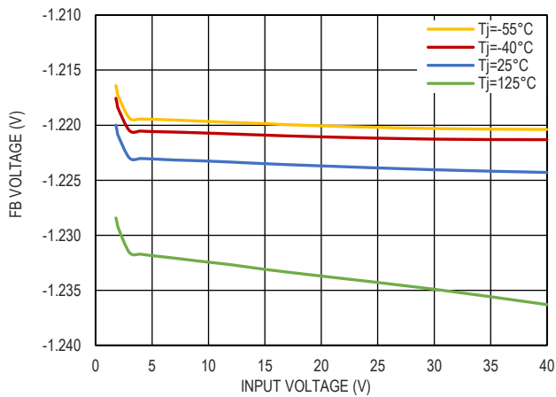
图 6. FB 引脚电压与输入电压的关系
