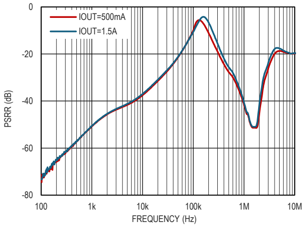
图 12. PSRR 和负载电流的关系, V_{OUT} = -4.3V , V_{IN} = -3.3V
