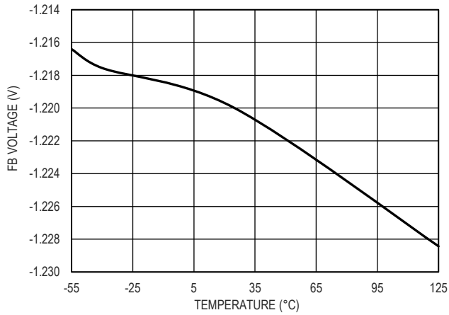
图 4. FB 引脚电压与结温 ( T_j ) 的关系
