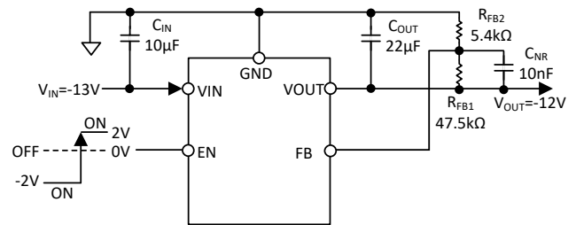
图 19. 更改可调输出 LDO 以降低噪声
