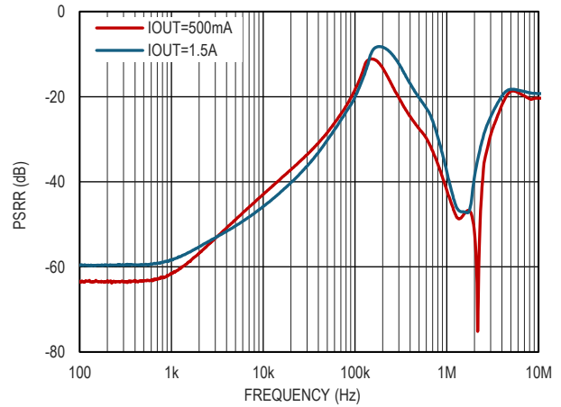
图 11. PSRR 和负载电流的关系, V_{OUT} = -3V , V_{IN} = -1.2V
