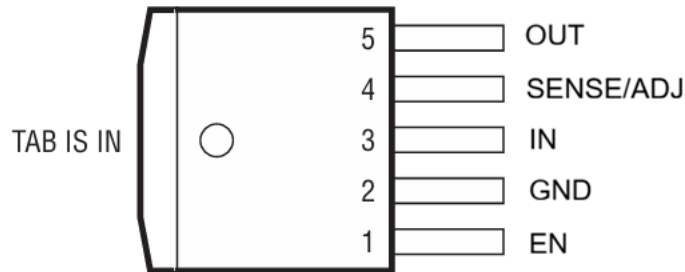
图 3. TO-263 引脚配置(顶视图)
