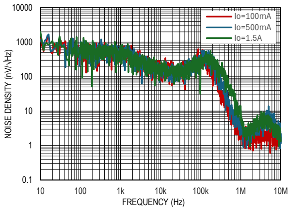
图 10. 噪声谱密度
