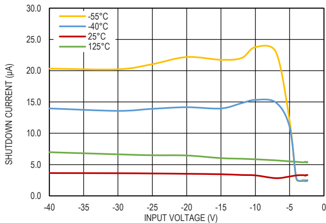
图 8. 关机电流与输入电压的关系
