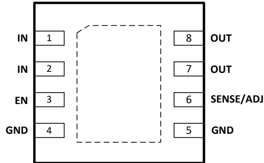
图 2. 3mm x 3mm DFN-8 引脚配置(顶视图)
