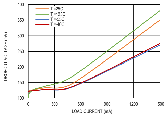
图 9. 压差电压和负载电流的关系
