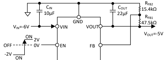
图 1 典型应用
