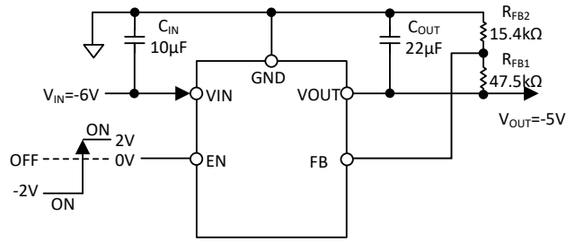
图 18. 设置可调输出电压
