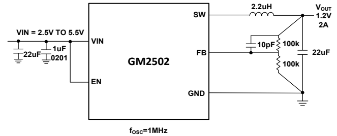
图 1. 1MHz 典型应用
