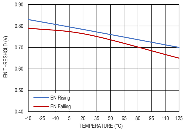
图 14. EN 阈值和温度的关系
