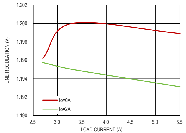
图 13. 输出电压线调整率, V_{OUT} = 1.2V
