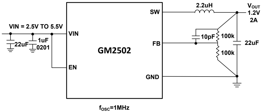
图 25. 1MHz, V_{IN}=3.3\text{V} , V_{OUT}=1.2\text{V} , I_{LOAD}=2\text{A}
