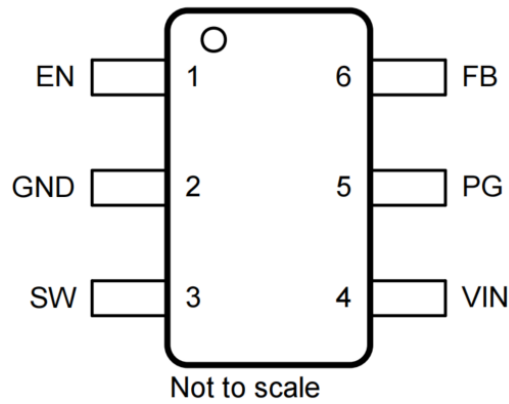
图 6.6 引脚 SOT-23 引脚配置
