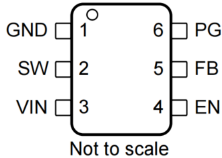
图 4.6 引脚 PSOT-563 (GM2502ARNZ--R7, 兼容 SOT-563) 引脚配置
