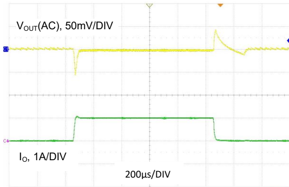
图 20. V_{OUT} = 1.2V , I_O = 0A 至 1A , 低功耗模式
