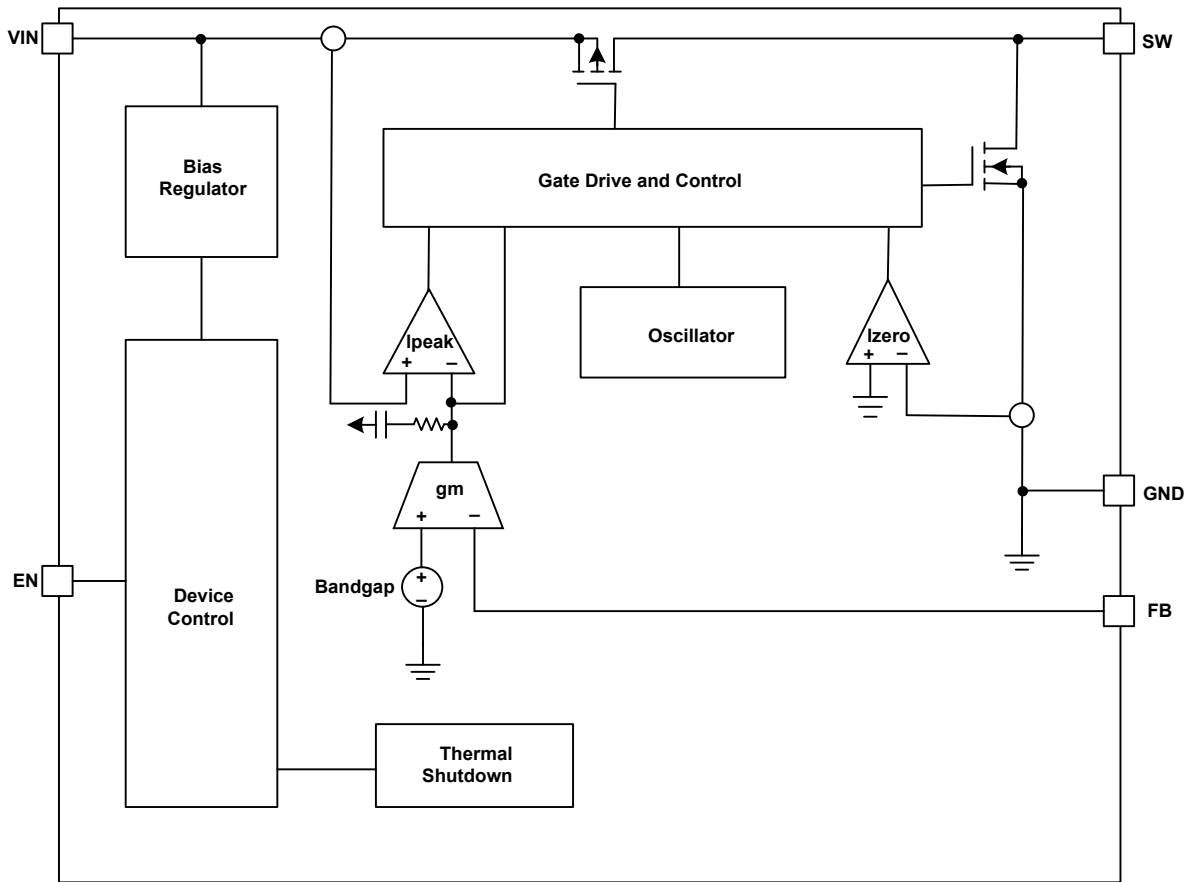
图 3 GM2502 功能框图
