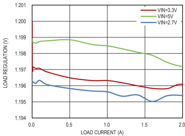
图 12. 输出电压负载调整率, V_{OUT} = 1.2V
