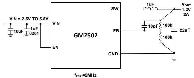
图 2. 2MHz 典型应用
