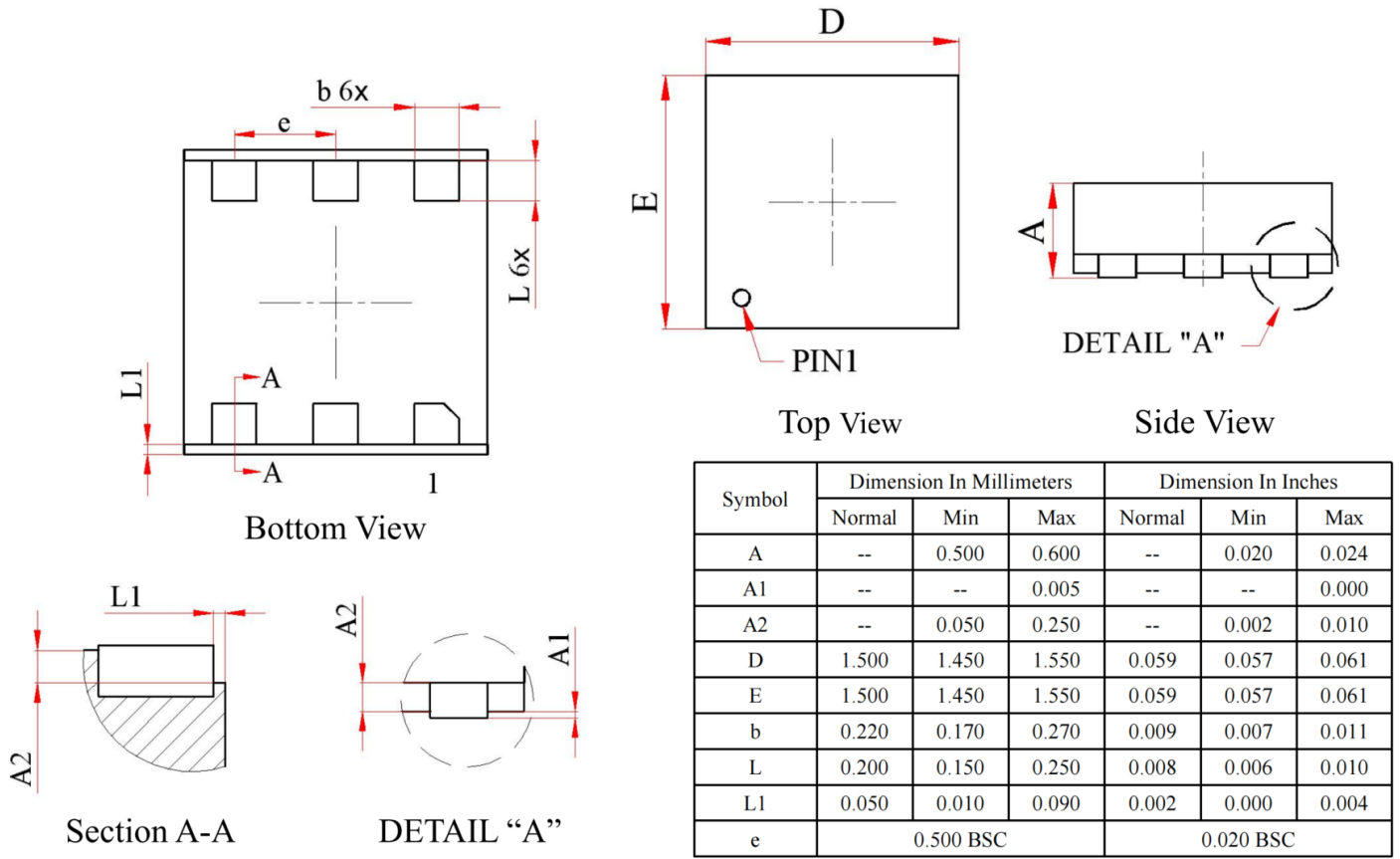
图 27. 6 引脚 PSOT-563
