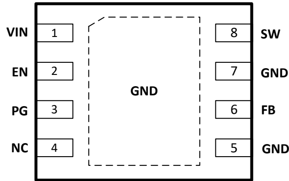
图 7.8 引脚 DFN 引脚配置
