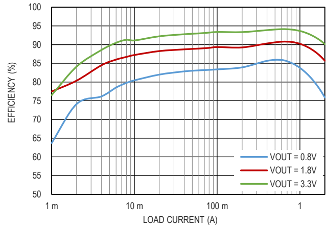
图 9. 效率曲线, V_{OUT} = 1.2V , F_{sw} = 1MHz
