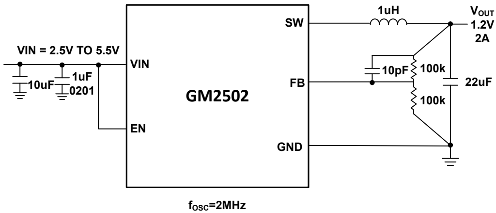
图 26. 2MHz, V_{IN}=3.3\text{V} , V_{OUT}=1.2\text{V} , I_{LOAD}=2\text{A}
