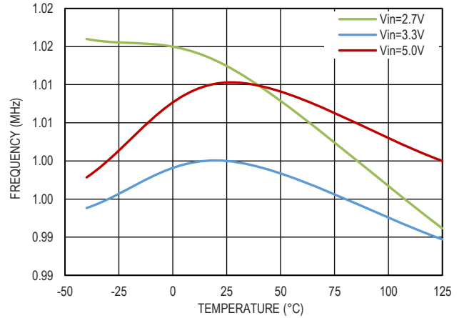
图 11. 频率和温度的关系
