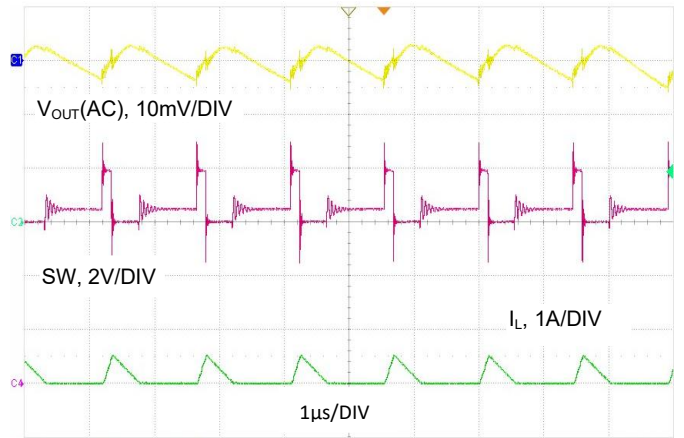
图 19. V_{OUT} = 1.2V , I_O = 100mA , 低功耗模式
