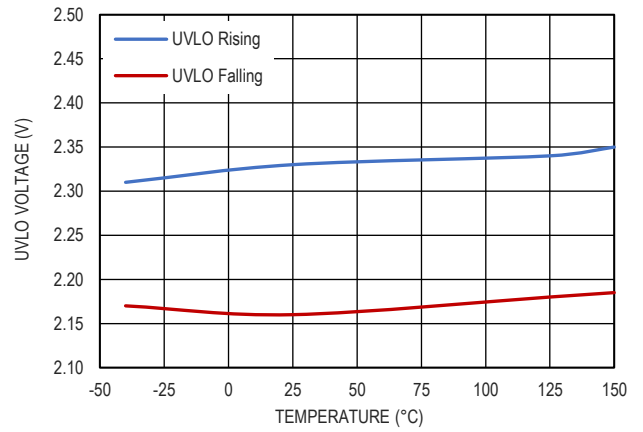
图 15. UVLO 阈值和温度的关系
