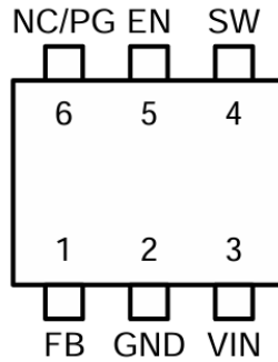
图 5.6 引脚 PSOT-563 (GM2502ARNZ-1-R7, 兼容 SOT-563) 引脚配置
