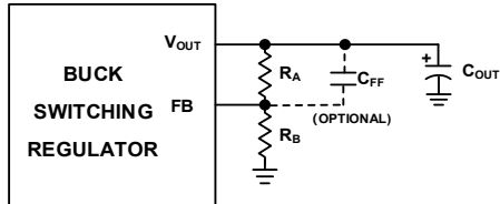
图 24. 反馈电阻网络
