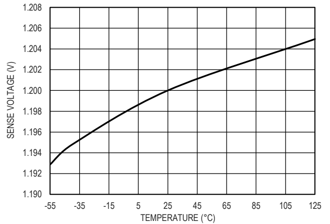
图 14. 1.2V FB 引脚电压精度
