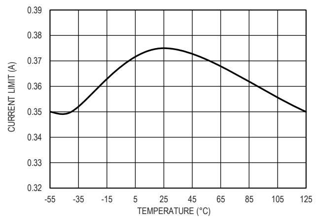
图 16. 输出限流值和温度的关系
