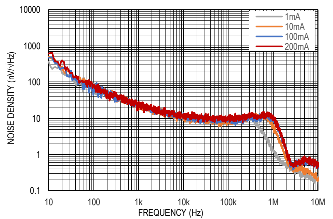
图 18. 输出噪声谱密度, V_{IN}=5\text{V} , V_{OUT}=3.6\text{V}
